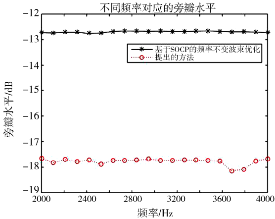
图 5 不同频率对应的波束旁瓣水平对比
