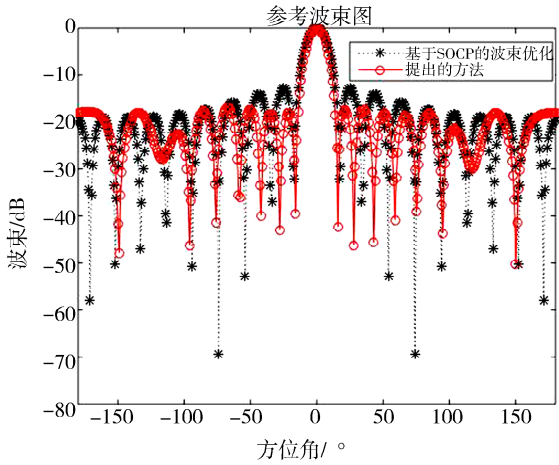
图 2 不同方法参考波束图 Fig. 2 Reference beam for different methods
