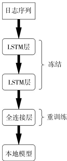
图 3 基于 LSTM 模型的迁移学习过程 Fig. 3 Transfer learning process based on LSTM
