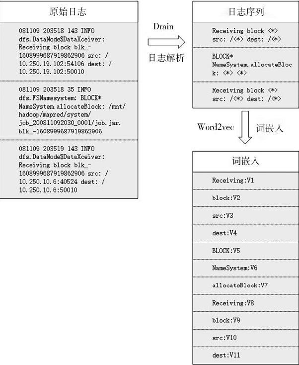
图 2 日志数据表征构建过程 Fig. 2 Logs representation construction process
